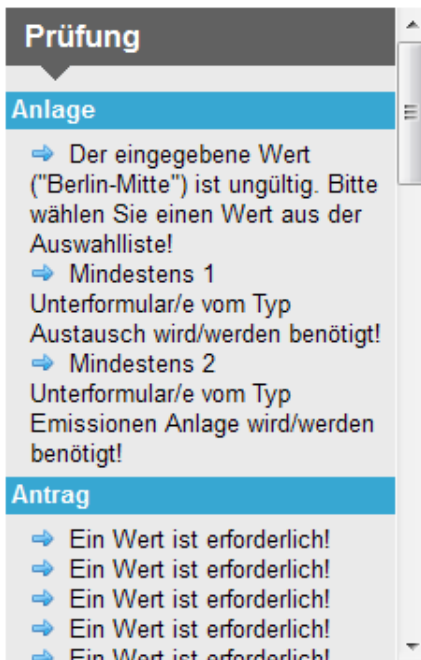
Abbildung 11: Prüfenster
