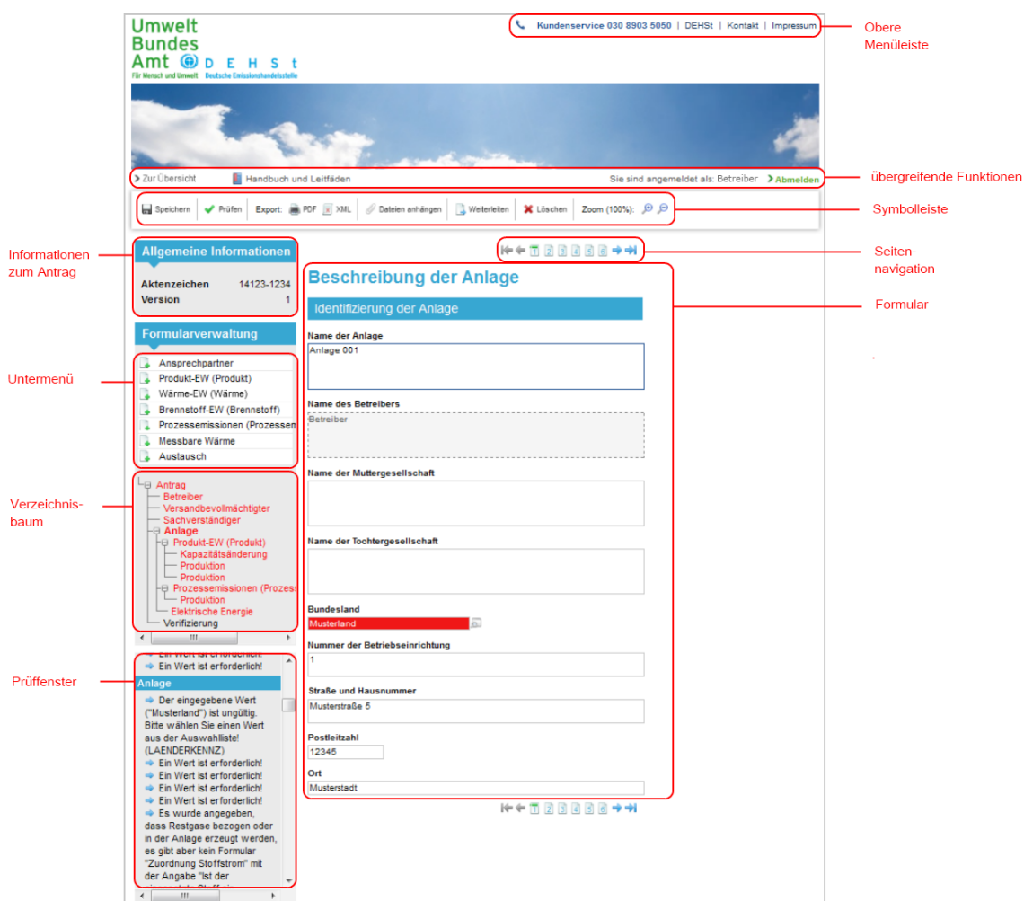
Abbildung 7: Zuteilungsantrag
