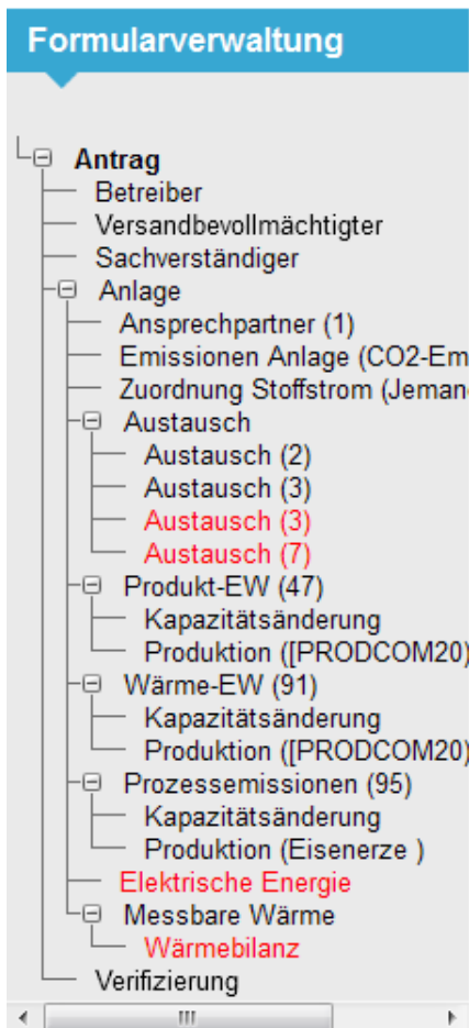
Abbildung 9: Verzeichnisbaum
